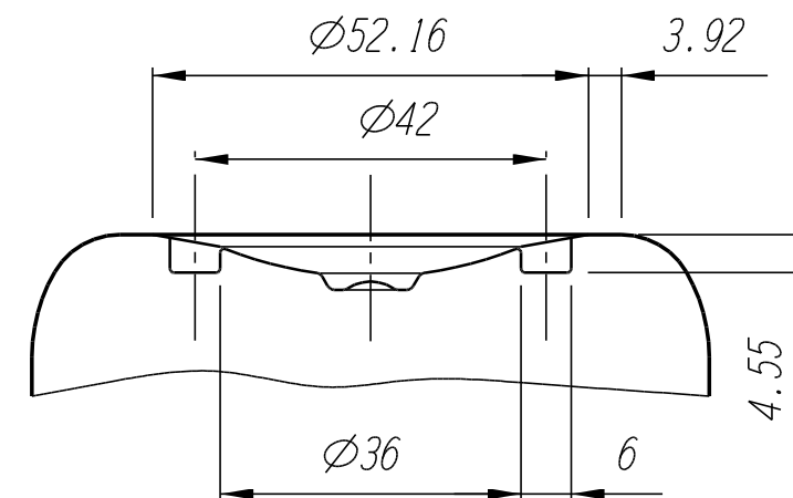
SEZIONE A-A
